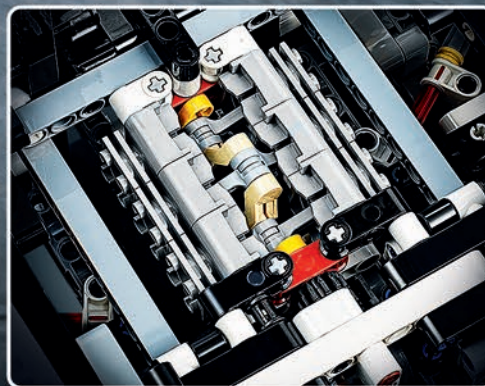
6-цилиндров двигател с движещи се бутала
